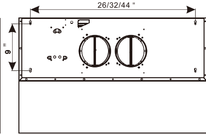
Model:KOS-30RH06H/KOS-36RH06H/KOS-48RH06H
