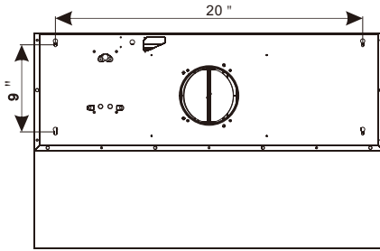
Model:KOS-24RH06H
